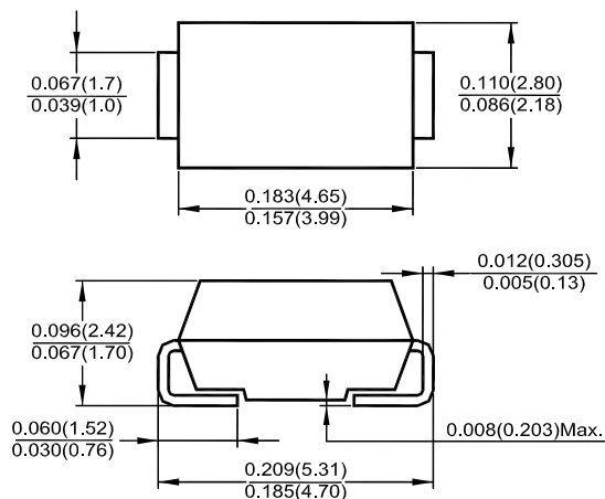
SMA (DO-214AC)
