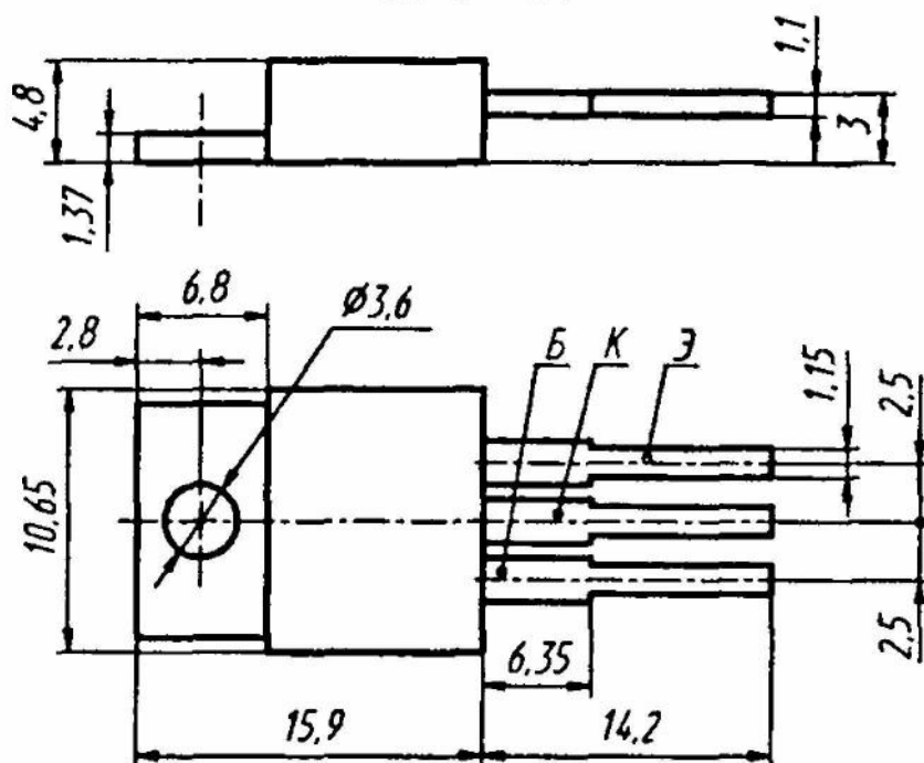
КТ851(А-В)
