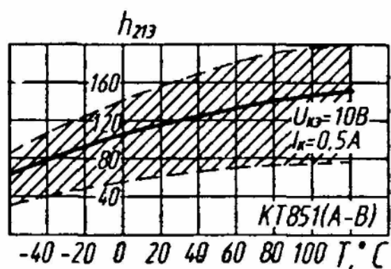
Зона возможных положений зависимости статического коэффициента передачи тока от температуры
