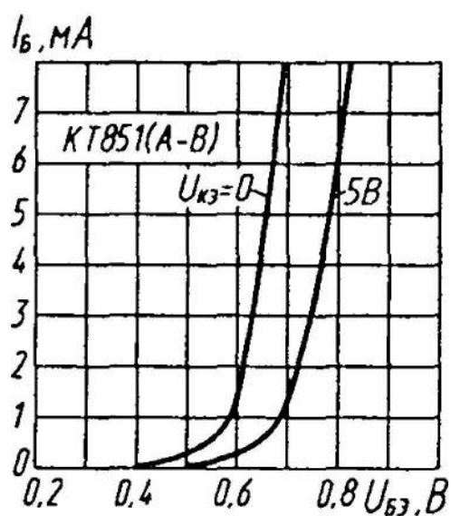
Входные характеристики
