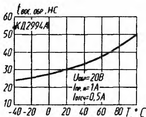
Зависимость времени обратного восстановления от температуры
