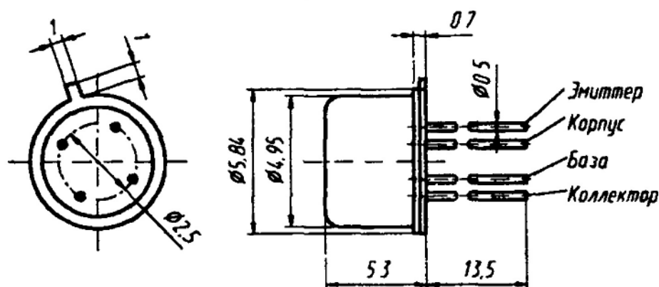
КТ368(АМ, БМ)
