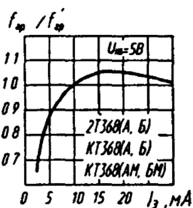
Зависимость граничной частоты от тока эмиттера
