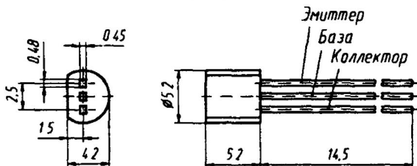
КТ368(АМ, БМ)
