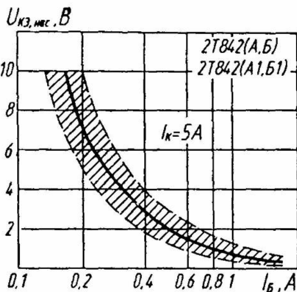
Зона возможных положений зависимости напряжения насыщения коллектор—эмиттер от тока базы
