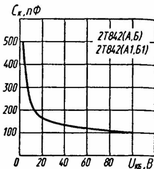
Зависимость емкости коллекторного перехода от напряжения коллектор—база
