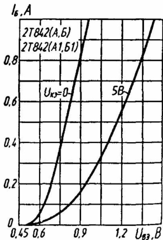
Входные характеристики
