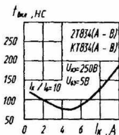
Зависимость времени включения от тока коллектора
