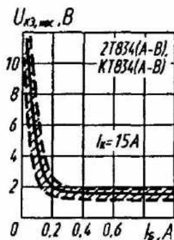
Зона возможных положений зависимости напряжения насыщения коллектор—эмиттер от тока базы
