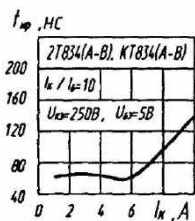
Зависимость времени нарастания от тока коллектора
