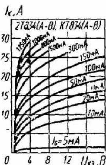
Выходные характеристики
