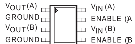
MIC5202-xxBM
