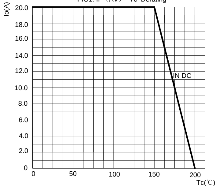
FIG1: IF (AV) --Tc Derating
