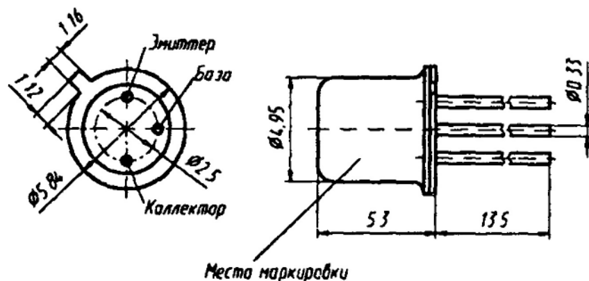
КТ3102(А-Д)
