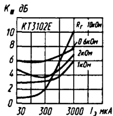
Зависимости коэффициента шума от тока эмиттера
