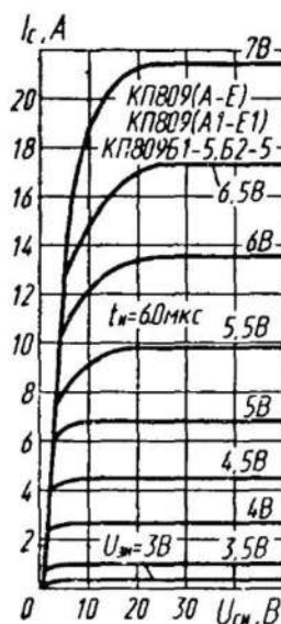
Выходные характеристики
