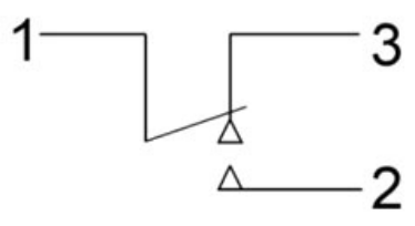
Коммутационная схема
