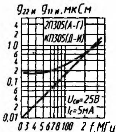
Зависимость активных входной и выходной проводимостей от частоты
