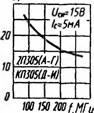
Зависимость коэффициента усиления от частоты
