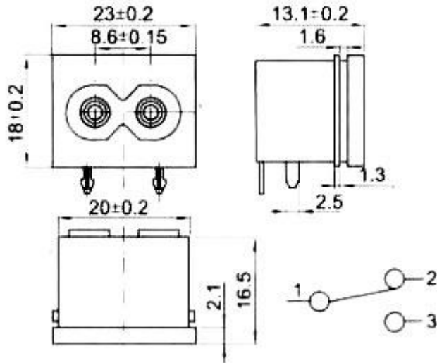
电源插座系列主要技术指标 Specification of Power socket
