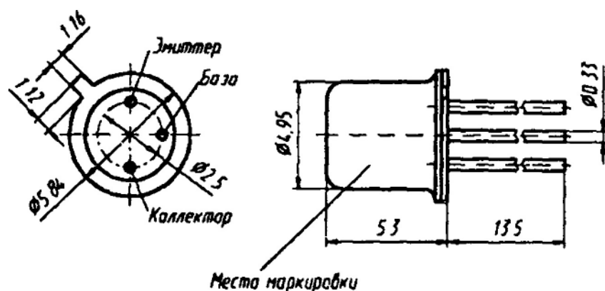
КТ3102(А-Д)
