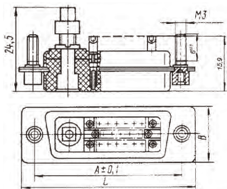
Розетка с в.ч контактами с фиксатором
