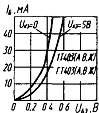
Входные характеристики
