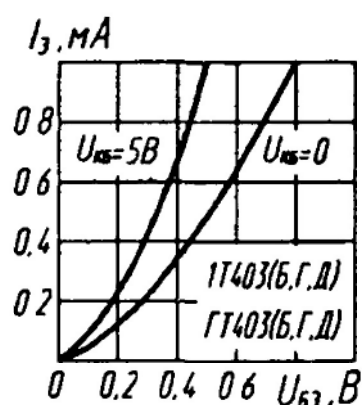
Зависимость тока эмиттера от напряжения база—эмиттер
