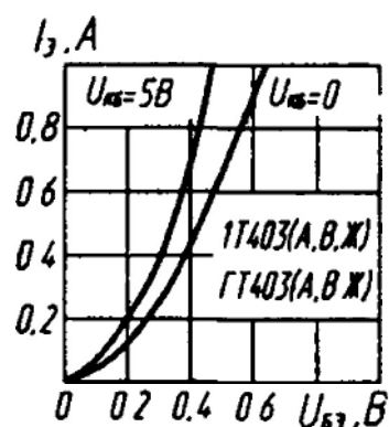
Зависимость тока эмиттера от напряжения база—эмиттер
