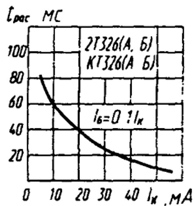
Зависимость времени рассасывания от тока коллектора
