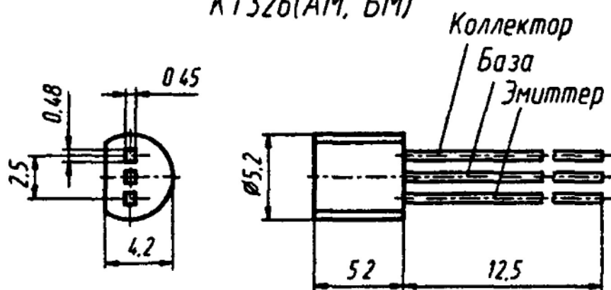
КТ326(АМ, БМ)
