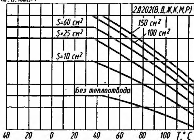
Зависимости допустимого прямого тока от температуры ( S — площадь теплоотвода)
