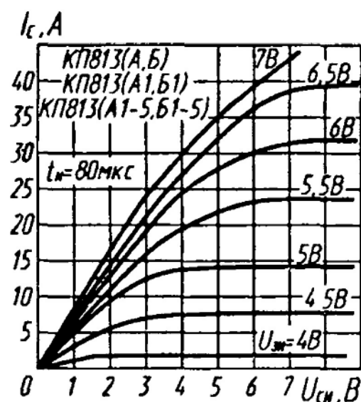
Выходные характеристики
