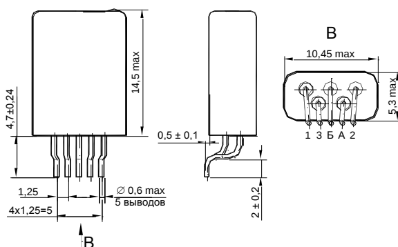
Рис. 2 - Общий вид реле РЭК63-1
