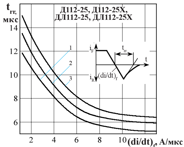
Рисунок 15 - Зависимость времени обратного восстановления t_{гр} от скорости спада прямого тока (di/dt)_f при температуре перехода T_{jm} = 150^\circ\text{C} , U_R = 100\text{ В} и при отношении амплитуды прямого тока I_F к допустимому среднему прямому току I_{F(AV)} равному: k = 0,5 (1); 1,0 (2); 1,5 (3); где k = I_F / I_{F(AV)} .
