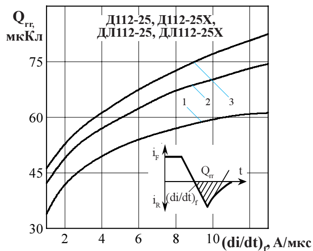
Рисунок 14 - Зависимость заряда восстановления Q_{гр} от скорости спада прямого тока (di/dt)_f при температуре перехода T_{jm} = 150^\circ\text{C} , U_R = 100\text{ В} и при отношении амплитуды прямого тока I_F к допустимому среднему прямому току I_{F(AV)} равному: k = 0,5 (1); 1,0 (2); 1,5 (3); где k = I_F / I_{F(AV)} .
