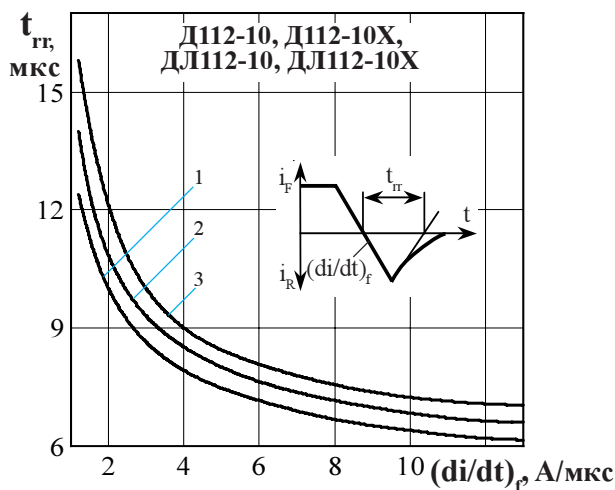
Рисунок 15 - Зависимость времени обратного восстановления t_{гр} от скорости спада прямого тока (di/dt)_f при температуре перехода T_{jm} = 150^\circ\text{C} , U_R = 100\text{ В} и при отношении амплитуды прямого тока I_F к допустимому среднему прямому току I_{F(AV)} равному: k = 0,5 (1); 1,0 (2); 1,5 (3); где k = I_F / I_{F(AV)} .
