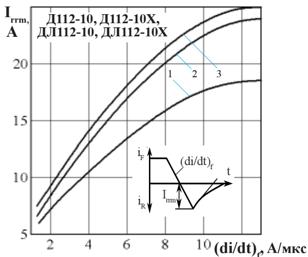
Рисунок 16 - Зависимость обратного тока восстановления I_{грм} от скорости спада прямого тока (di/dt)_f при температуре перехода T_{jm} = 150^\circ\text{C} , U_R = 100\text{ В} и при отношении амплитуды прямого тока I_F к допустимому среднему прямому току I_{F(AV)} равному: k = 0,5 (1); 1,0 (2); 1,5 (3); где k = I_F / I_{F(AV)} .
