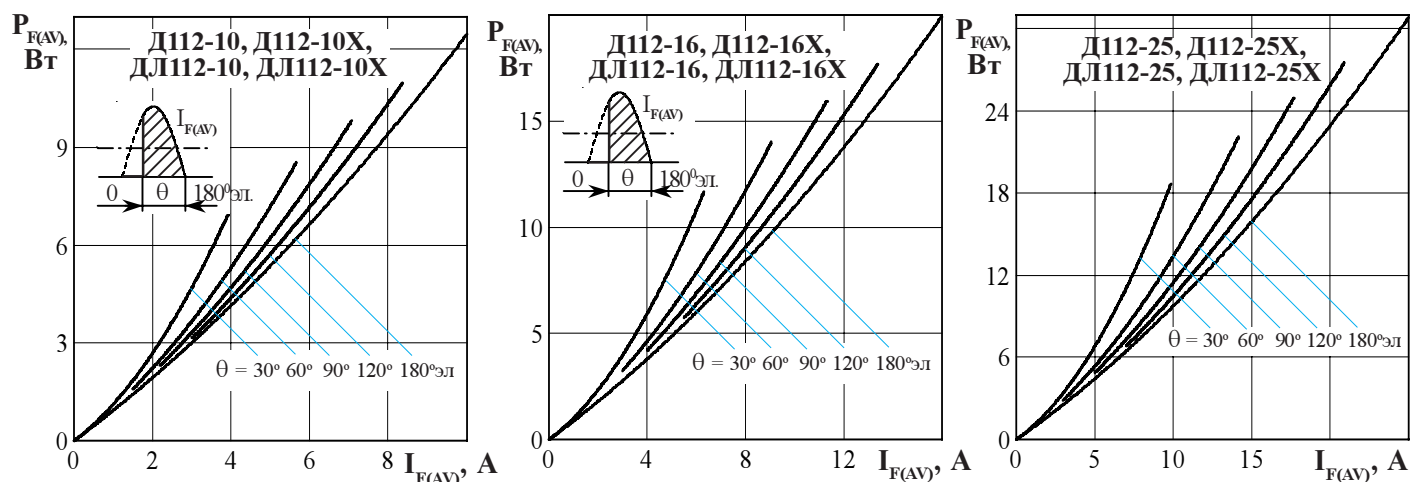
Рисунок 6 - Зависимость средней прямой рассеиваемой мощности P_{F(AV)} от среднего прямого тока I_{F(AV)} синусоидальной формы частотой f = 50 Гц
