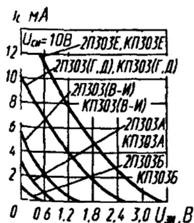
Проходные характеристики
